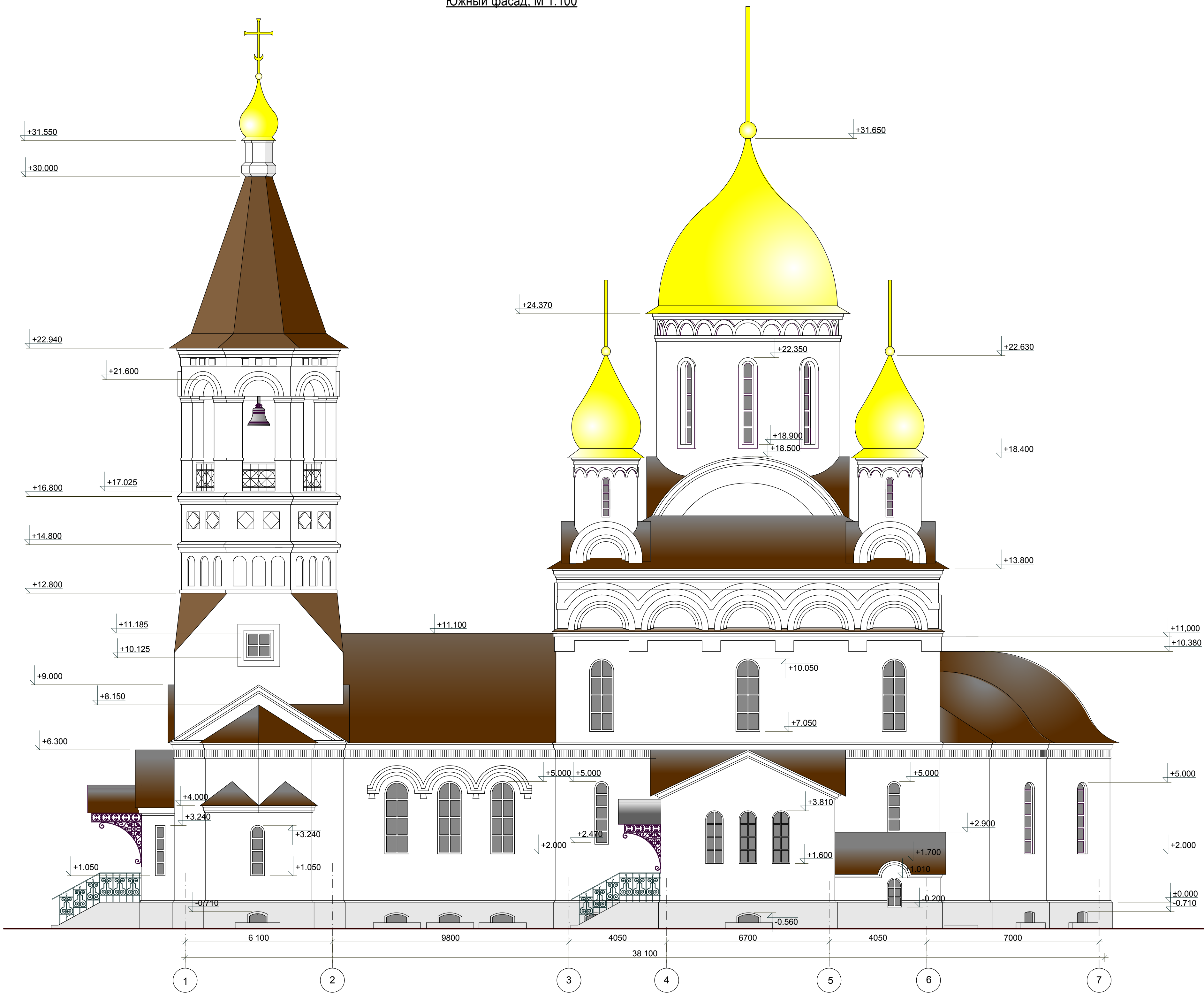
Южный фасад, М 1:100
